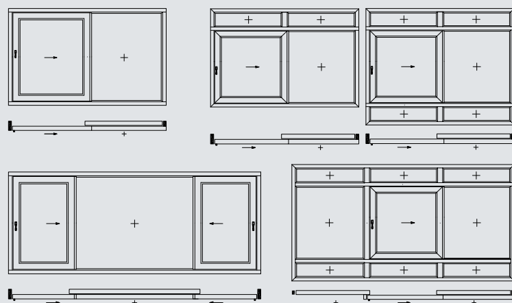
Sheme otvaranja kliznih stijena PreMiSlide 76
